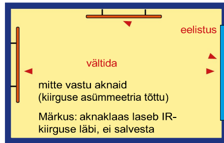
Joonis. Lisaküttekeha paigutamine ühe aknaga ruumi
