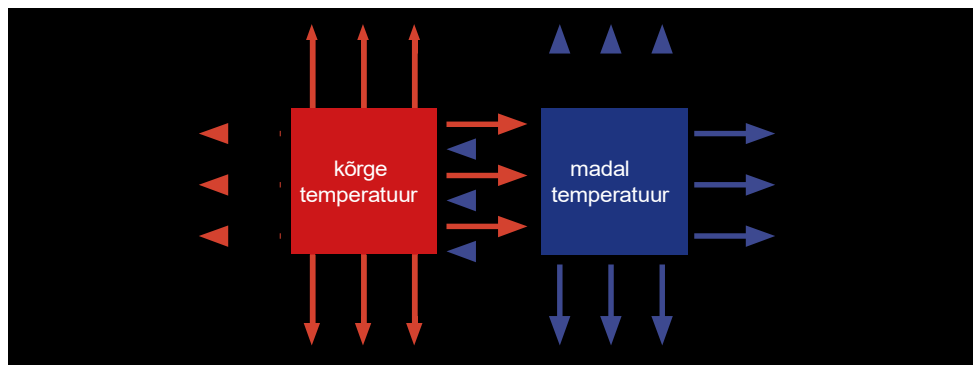
Joonis. Kahe keha vaheline kiirgus
